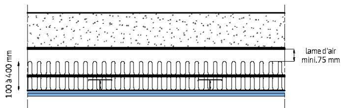
Lame d'air : Cas avec isolant
