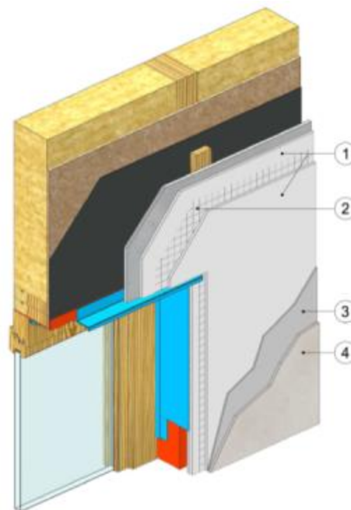
Figure 33 - COB- Perspective linteau - Traitement des menuiseries (Pose tunnel intérieur) Etape 4 - Traitement des joints et têtes de vis
