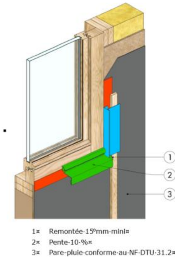
Figure 38 - COB - Perspective appuis - Traitement des menuiseries (Pose tunnel extérieur)
