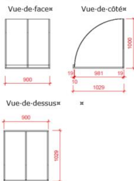
Figure 42 - Exemple de gabarit pour le pré-cintrage des plaques AQUAPANEL® avant mise en œuvre
