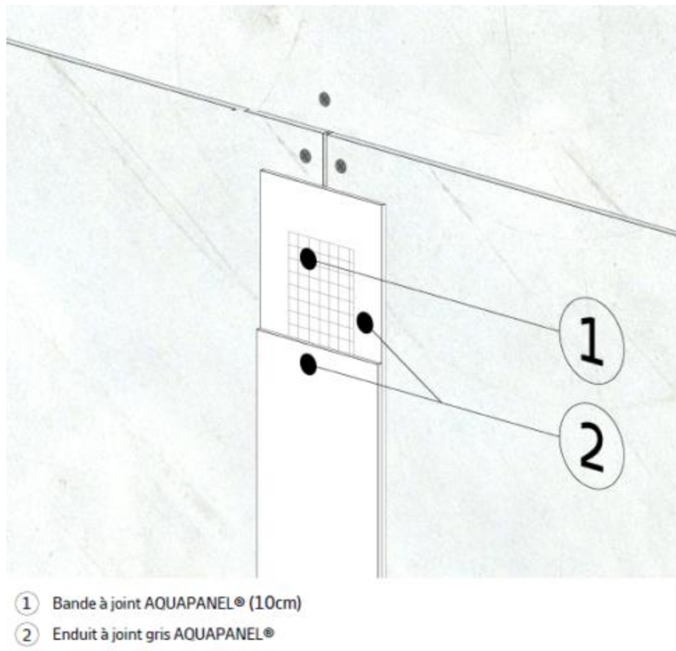
Figure 10 - Traitement des joints entre plaques
