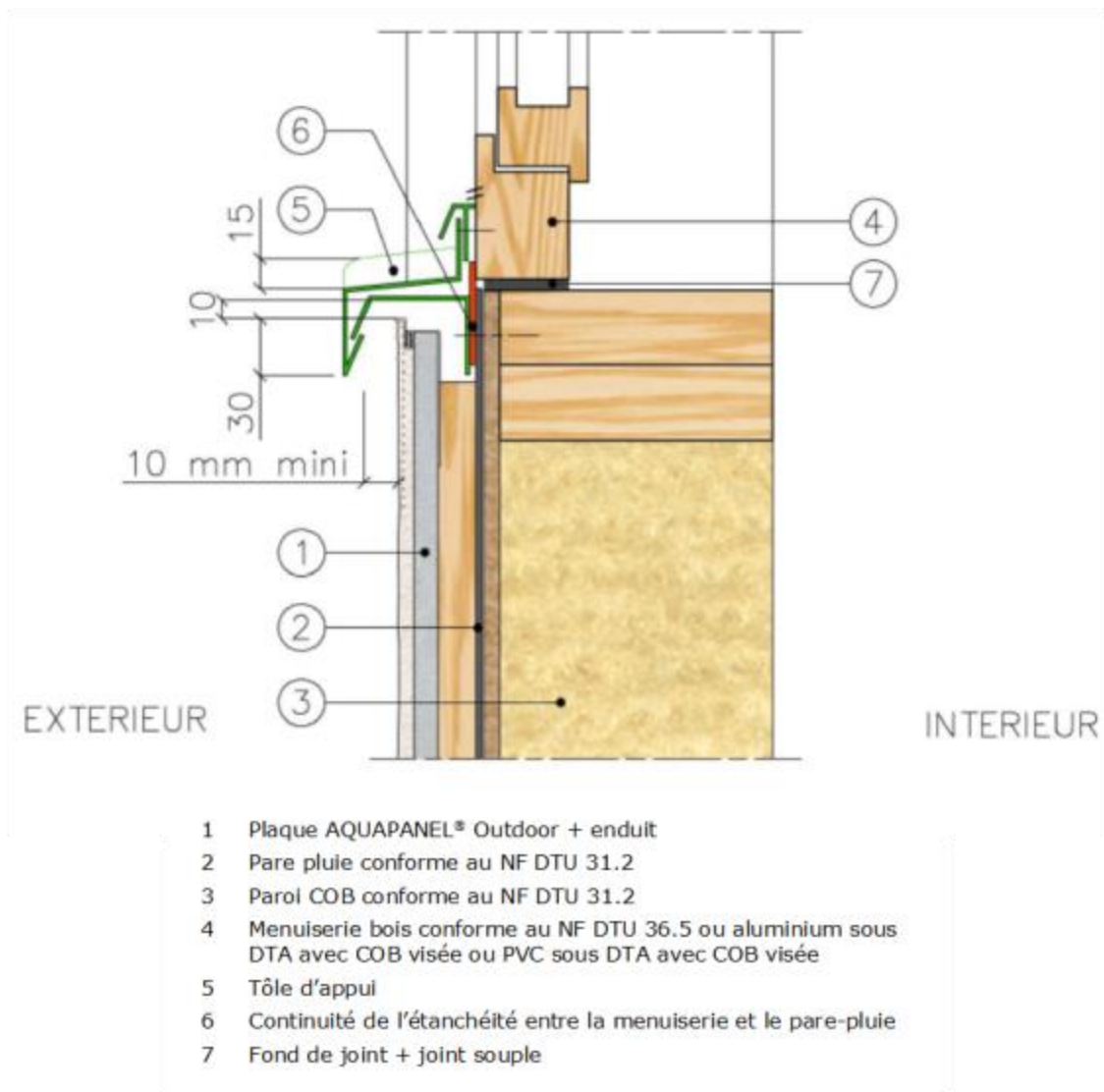
Figure 35 - COB - Coupe sur appui - Traitement des menuiseries (Pose tunnel extérieur)
