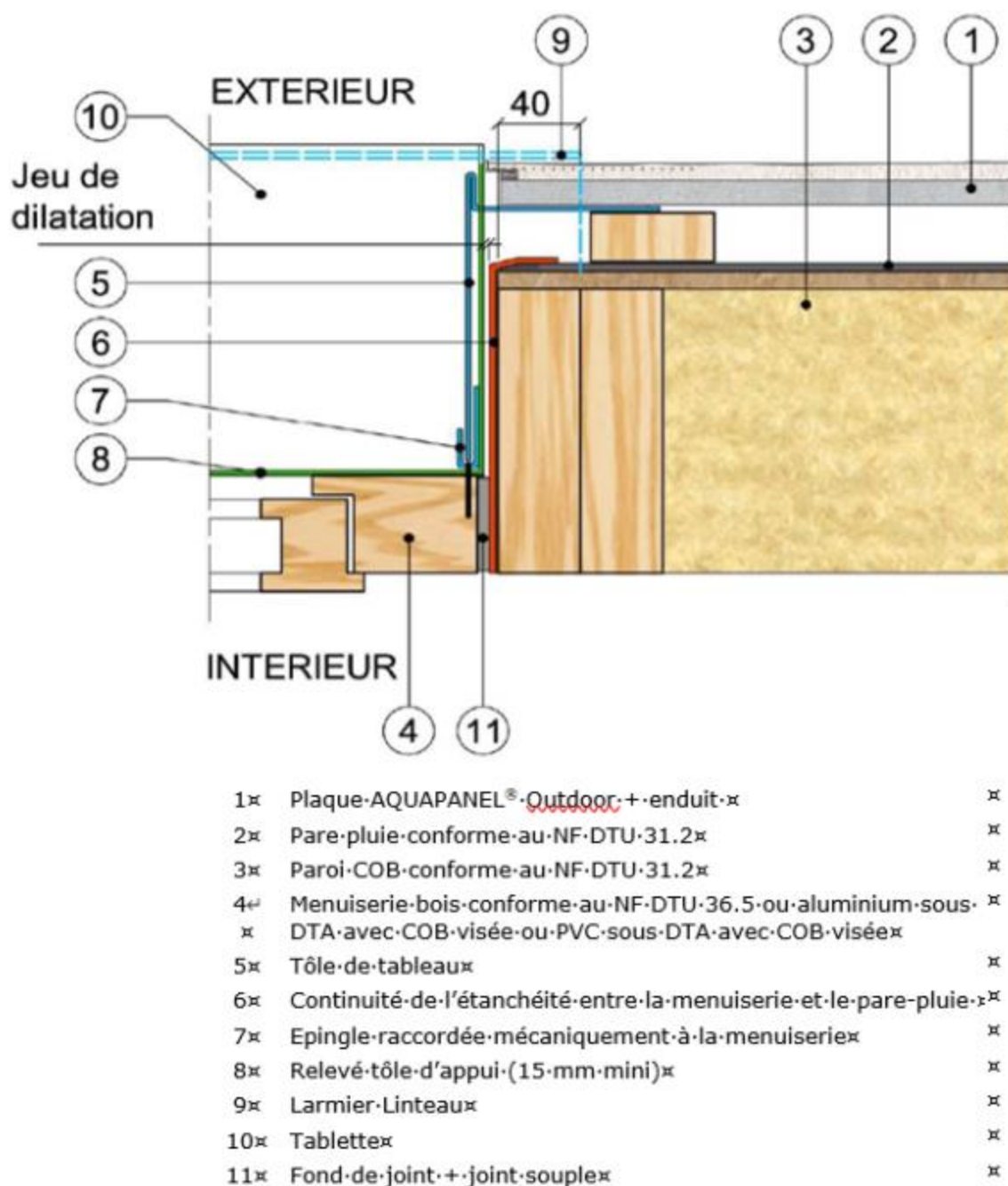
Figure 26 - COB – Coupe sur tableau de baie - Dispositions particulières du traitement des baies (menuiserie en tunnel intérieur)
