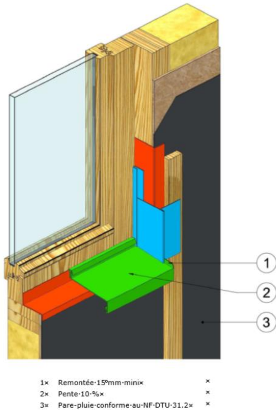
Figure 28 - COB – Perspective appui de baie - Dispositions particulières du traitement des baies (menuiserie en tunnel intérieur)
