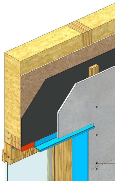
Figure 29 - COB - Perspective linteau - Traitement des menuiseries (Pose tunnel intérieur) Etape 1 – solin avec larmier
