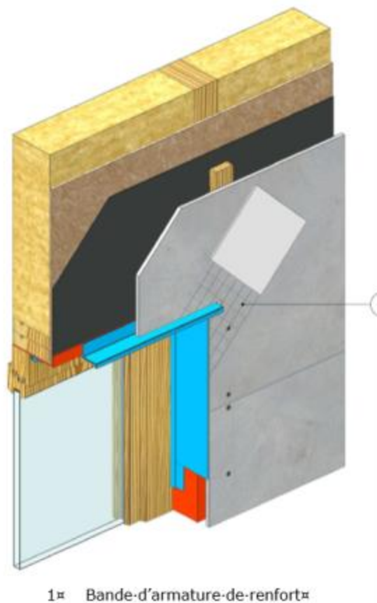
Figure 32 - COB- Perspective linteau - Traitement des menuiseries (Pose tunnel intérieur) Etape 3 - Renforcement des ouvertures
