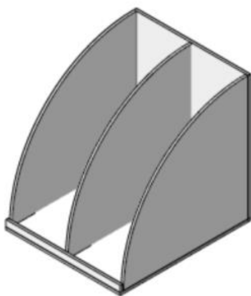
Figure 42 - Exemple de gabarit pour le pré-cintrage des plaques AQUAPANEL® avant mise en œuvre
