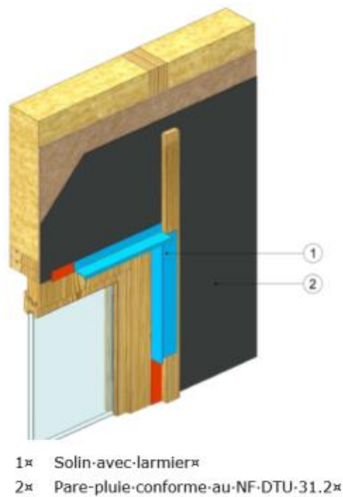
Figure 39 - COB - Perspective linteau - Traitement des menuiseries (Pose tunnel extérieur) Solin avec larmier
