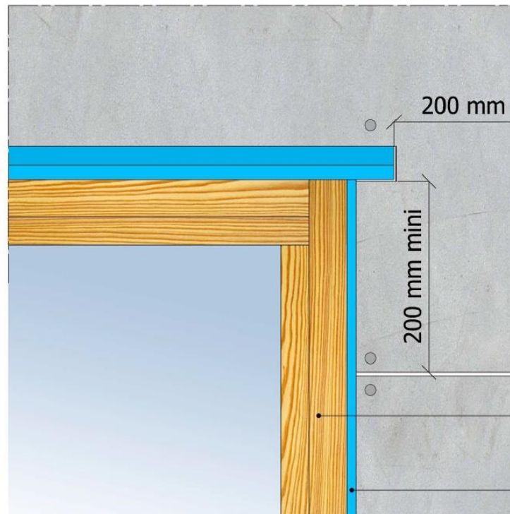
Figure 31 - COB --Perspective linteau - Traitement des menuiseries (Pose tunnel intérieur ou extérieur) Etape 2 - Détail d'angle
