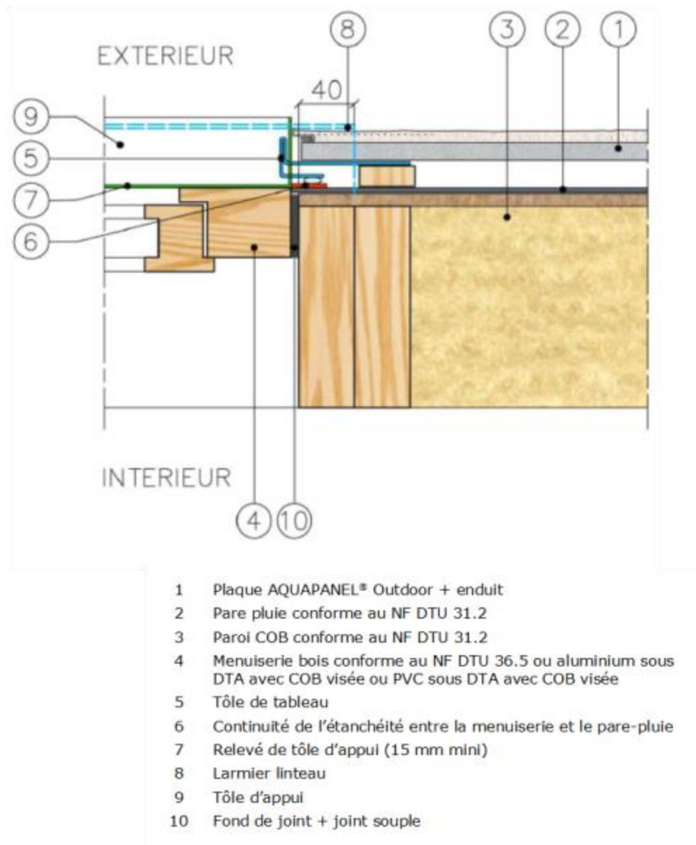
Figure 36 - COB - Coupe sur tableau - Traitement des menuiseries (Pose tunnel extérieur)
