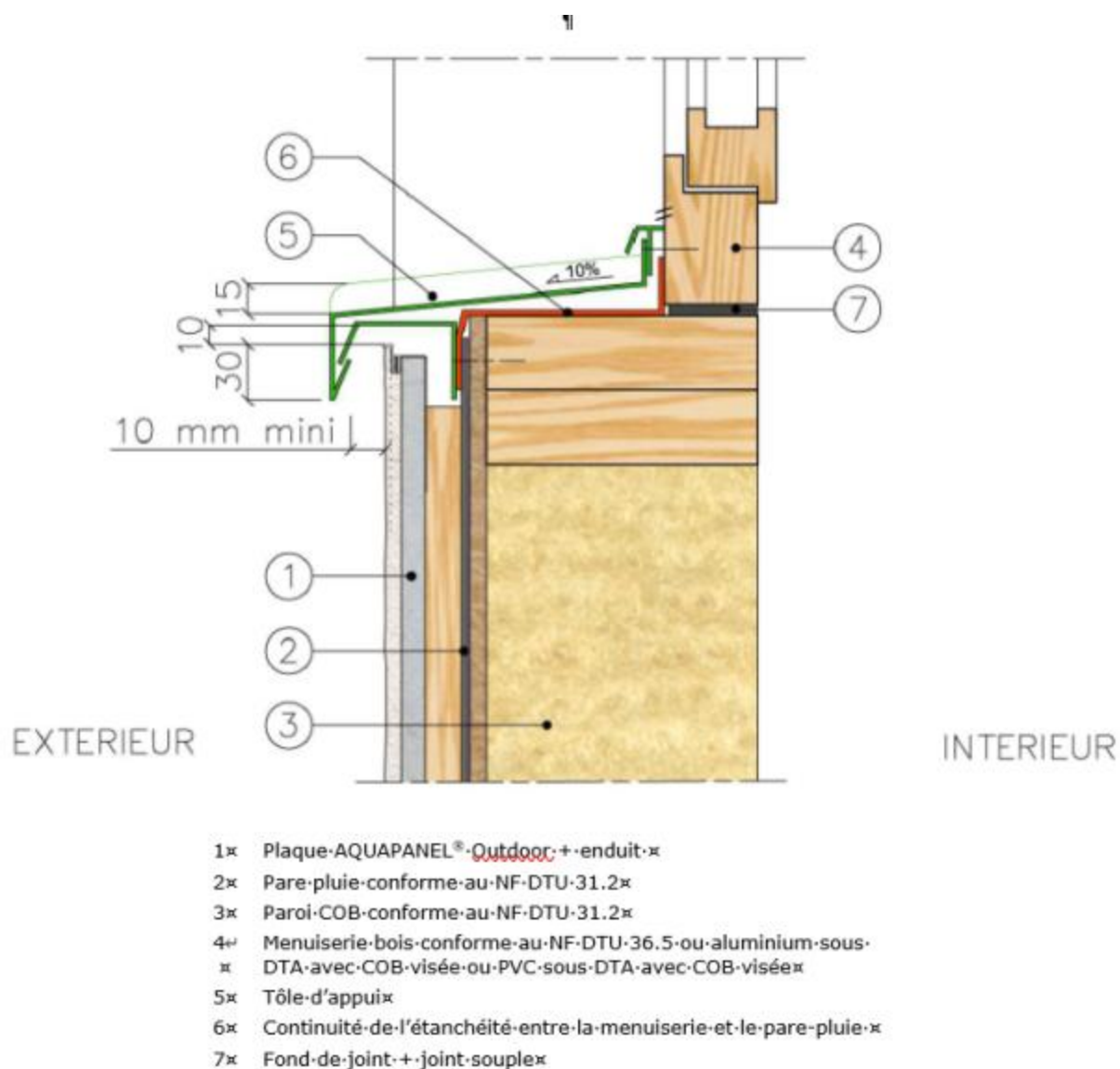
Figure 25 - COB – Coupe sur appui de baie - Dispositions particulières du traitement des baies (menuiserie en tunnel intérieur)
