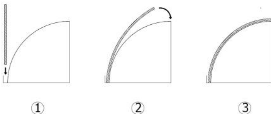
Figure 43 - Pré-cintrage de la plaque
