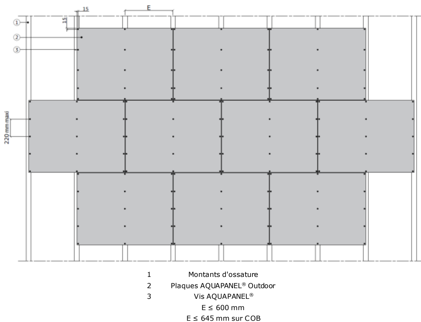
Figure 8 - Calepinage des plaques et espacement des vis - pose horizontale
