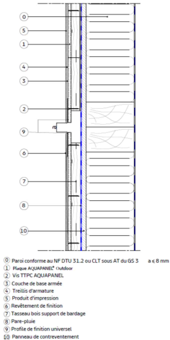
Figure 15 - COB, CLT - Joint de fractionnement horizontal ouvert au droit d'un plancher en situation a, b, c, d < 6 m et en situation a, b, c < 10 m - Ossatures bois sur COB
