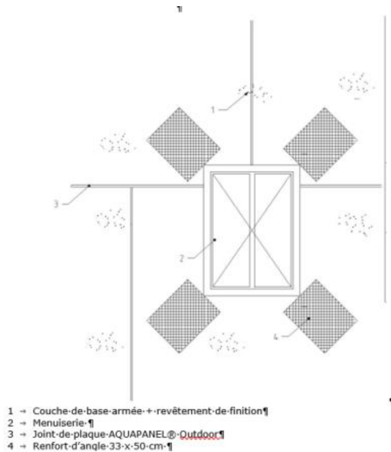
Figure 24 - Mise en œuvre des mouchoirs aux angles des ouvertures
